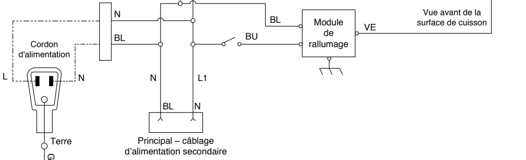
Schéma de la table de cuisson à 6 brûleurs
