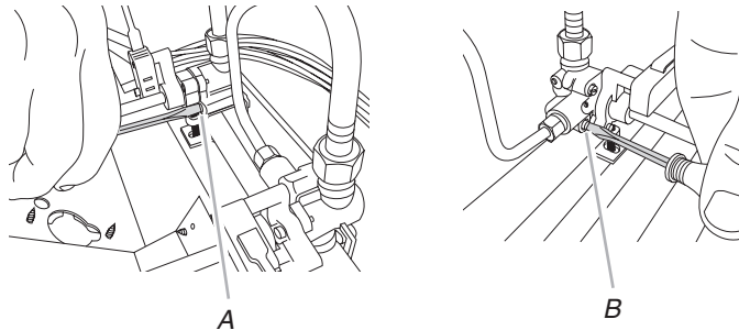
A. Tornillo de ajuste del quemador de una llama (en la parte derecha de la válvula)
