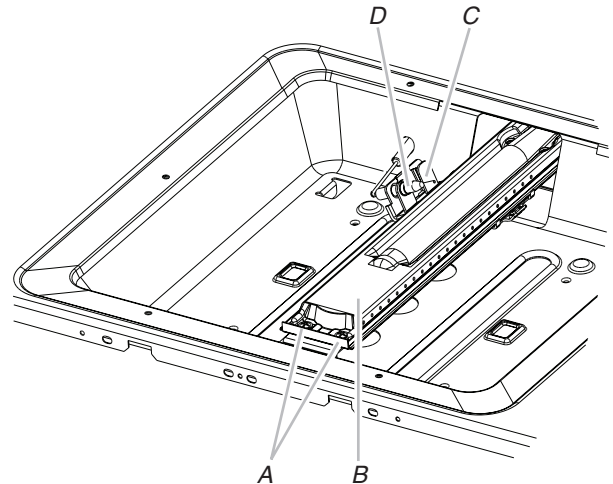
A. Vis du brûleur de cuisson au four B. Brûleur de cuisson au four C. Support de l'électrode du brûleur de cuisson au four D. Electrode du brûleur de cuisson au four
