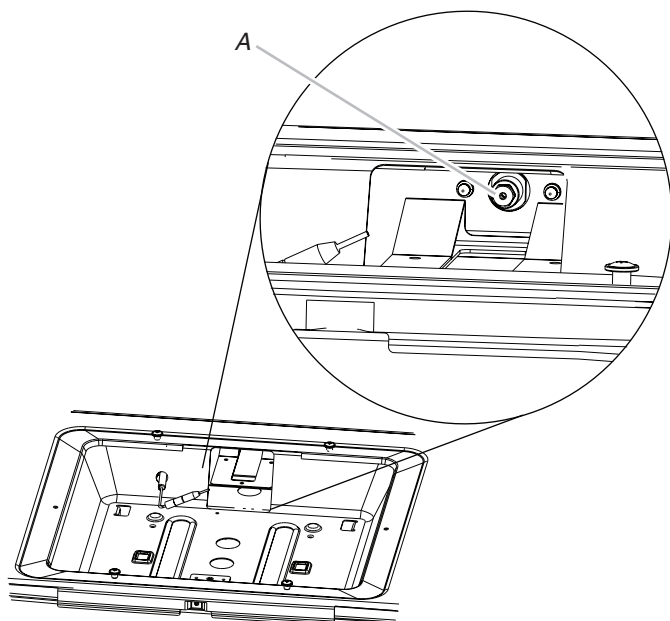
A. Tornillo del orificio de gas
