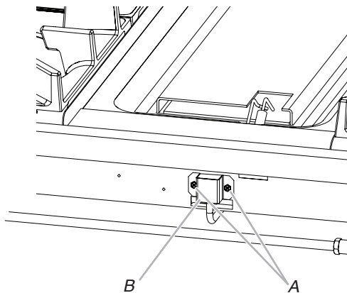
A. Tornillos B. Soporte del orificio de la parrilla
