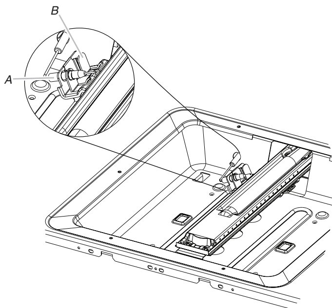
A. Electrodo del quemador para hornear del horno B. Soporte del electrodo del quemador para hornear del horno
