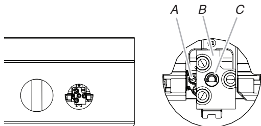
A. Tornillo de ajuste bajo-reducción de fuego lento B. Interrupción de ignición C. Tornillo de ajuste bajo-reducción principal
