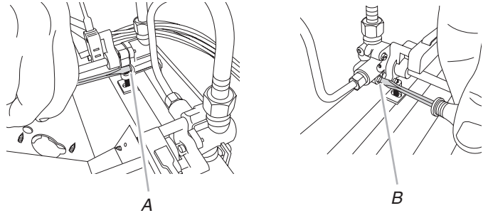
A. Vis de réglage du brûleur à flamme simple (du côté droit du robinet)
