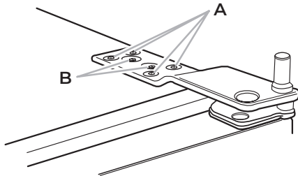
A. Vis de montage à tête plate Torx 27 B. Vis de montage à tête hexagonale de 1/4 po
