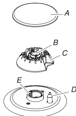
A. Chapeau de brûleur B. Tube d'arrivée de gaz C. Base du brûleur D. Électrode d'allumage E. Support d'injecteur à orifice
