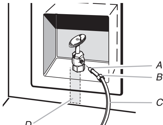
A. Manguito B. Tuerca C. Tubería de cobre (al refrigerador) D. Línea de suministro de la casa (1/2" como mínimo)
