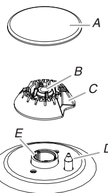
C. Base du brûleur
